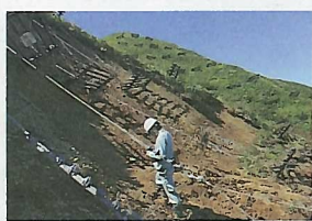
礼文島での豪雨による崩壊斜面の調査
